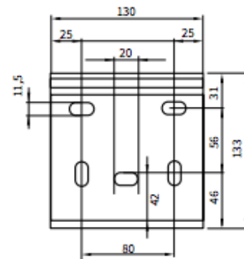
Vooraanzicht muursteun wandmontage
