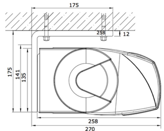
Plafondmontage
