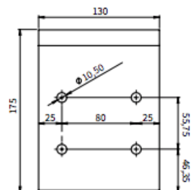
Vooraanzicht plafondsteun
